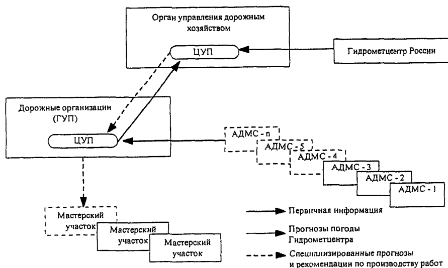
Рис. 3.1. Примерная схема получения и передачи информации о погодных условиях на автодороге
